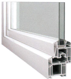
Inoutic Arcade - egyenes szárny
